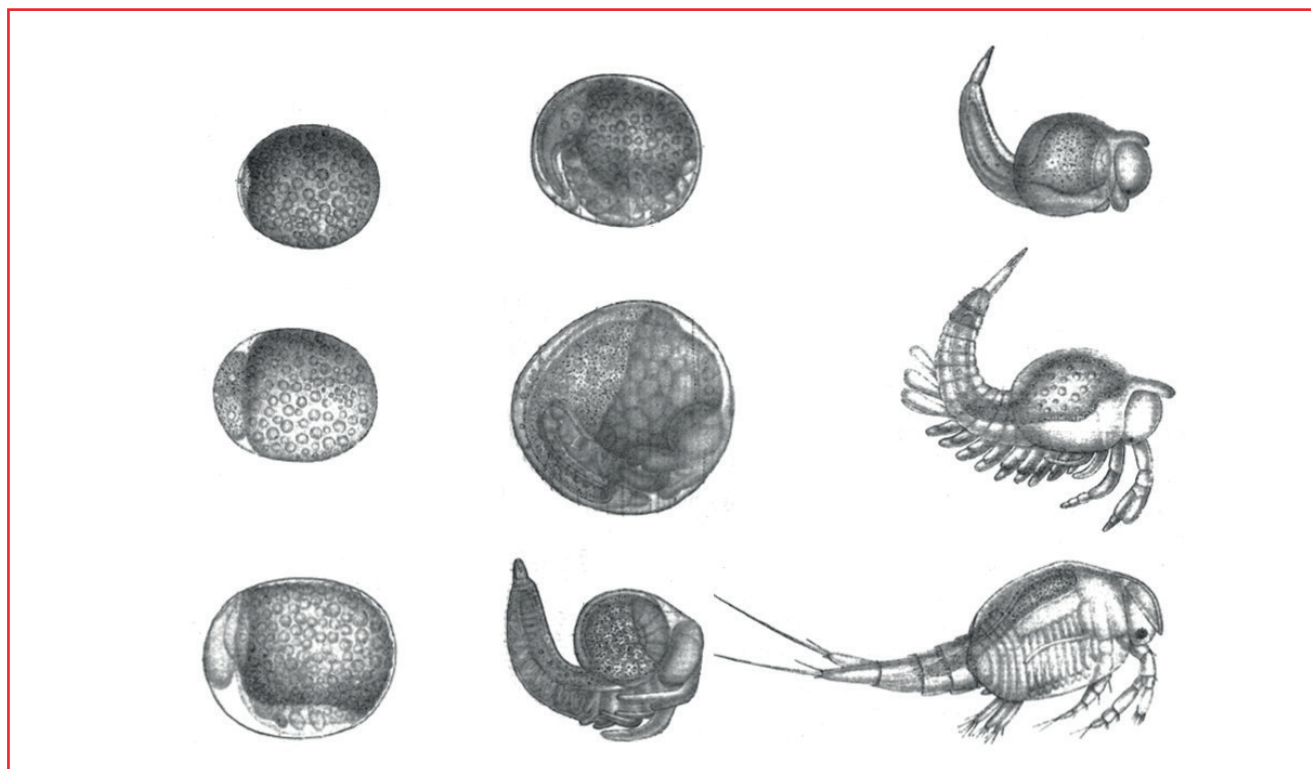
Fig. 1 - Histoire du développement de Nebalia geoffroy (d'après [6]). Stades de développement depuis l'œuf fécondé (en haut, à gauche) jusqu'au crustacé adulte (en bas, à droite).
